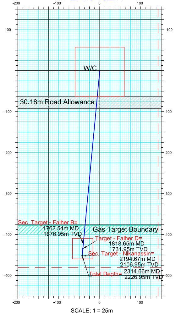
SCALE: 1 = 25m
